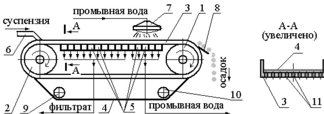
Рис. 10.5 – Ленточный вакуум-фильтр:
