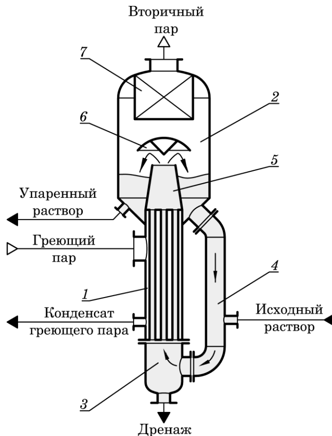
Рис. 13.8 – Вертикальный трубчатый аппарат с соосной греющей камерой, естественной циркуляцией раствора и вынесенной зоной кипения: 1 – греющая камера; 2 – сепаратор; 3 – нижняя крышка (днище) греющей камеры; 4 – циркуляционная труба; 5 – труба вскипания; 6 – отбойник; 7 – каплеотделитель
