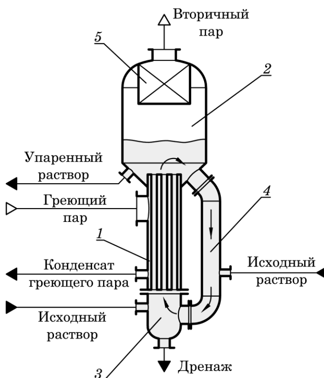
Рис. 13.6 – Вертикальный трубчатый выпарной аппарат с соосной греющей камерой и вынесенной циркуляционной трубой: 1 – греющая камера; 2 – сепаратор; 3 – нижняя крышка (днище) греющей камеры; 4 – циркуляционная труба; 5 – каплеотделитель
