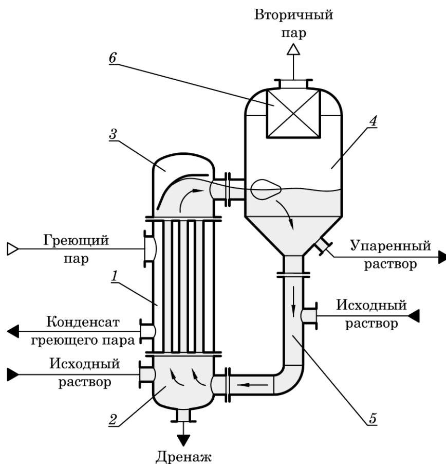
Рис. 13.7 – Выпарной аппарат с вынесенной греющей камерой: 1 – греющая камера; 2 – нижняя крышка (днище) греющей камеры; 3 – верхняя крышка греющей камеры; 4 – сепаратор; 5 – циркуляционная труба; 6 – каплеотделитель
