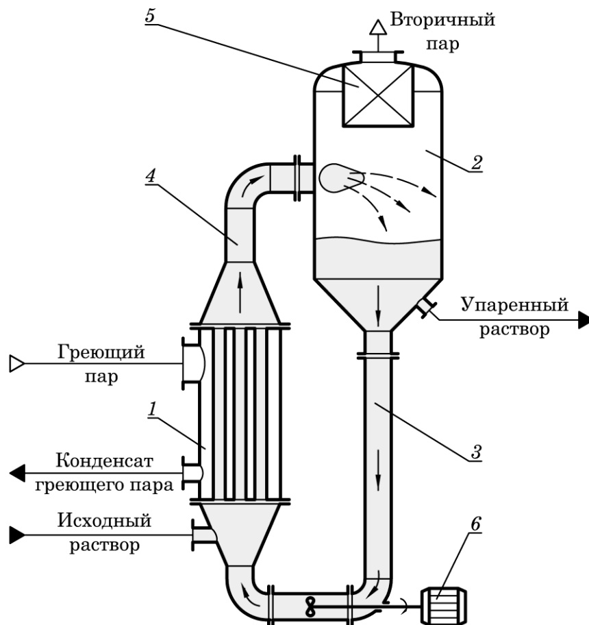
Рис. 13.9 – Вертикальный трубчатый аппарат с вынесенной греющей камерой и принудительной циркуляцией раствора:
