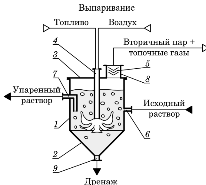
Рис. 13.11 – Выпарной аппарат с погружной горелкой: 1 – корпус; 2 – днище; 3 – крышка; 4 – погружная горелка; 5 – каплеотделитель; 6–9 – штуцера
