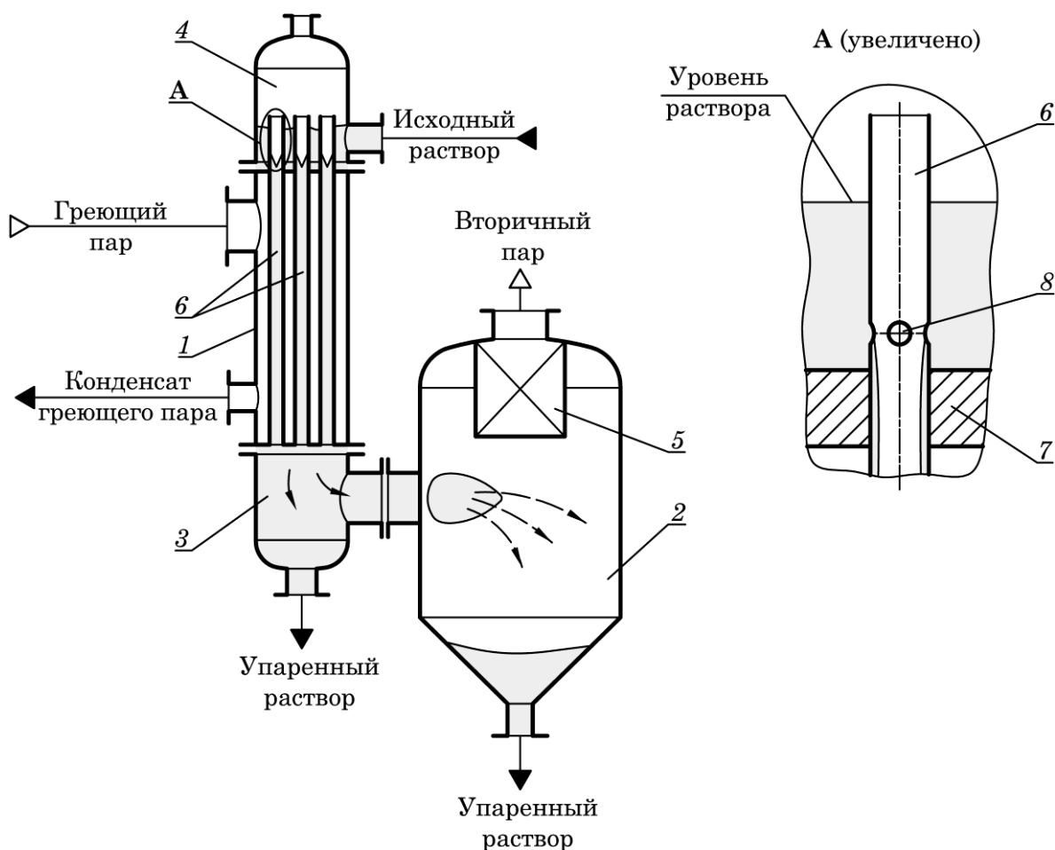
Рис. 13.10 – Вертикальный трубчатый аппарат со стекающей пленкой раствора: 1 – греющая камера; 2 – сепаратор; 3 – нижняя крышка (днище) греющей камеры; 4 – верхняя крышка греющей камеры; 5 – каплеотделитель; 6 – кипяtilьные трубы; 7 – верхняя трубная решетка; 8 – калиброванные отверстия
