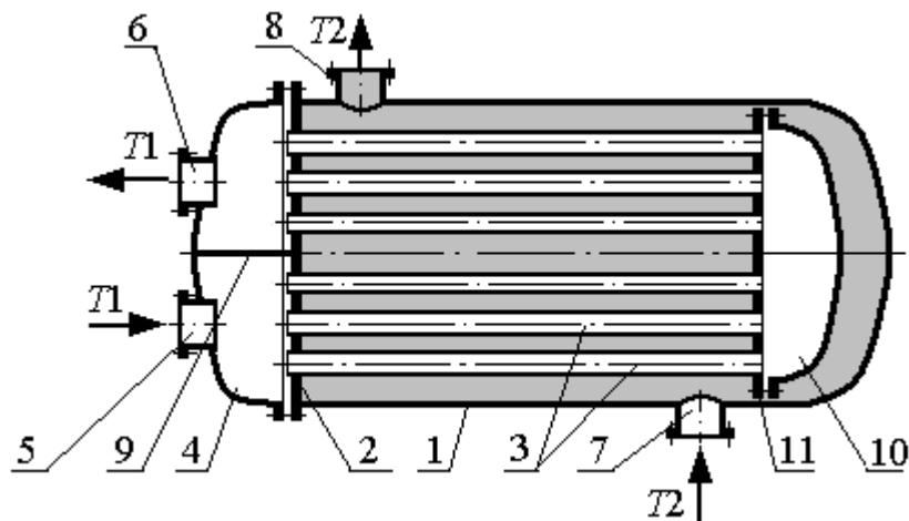
Рис. 4 – Кожухотрубчатый теплообменник с плавающей головой: 1 – кожух; 2 – трубная решетка; 3 – трубы; 4 – крышка; 5 и 6 – штуцера трубного пространства; 7 и 8 – штуцера межтрубного пространства; 9 – перегородка в распределительной камере; 10 – крышка плавающей головы; 11 – трубная решетка плавающей головы
