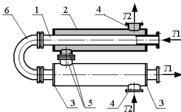
Рис. 5 – Двухтрубный секционный теплообменник:
