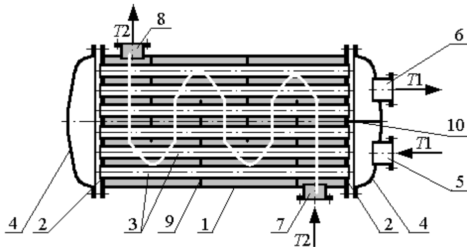
Рис. 2 – Многоходовой по трубному и межтрубному пространству кожухотрубчатый теплообменник:
