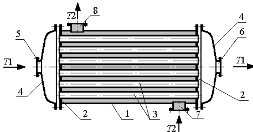
Рис. 1 – Одноходовой кожухотрубчатый теплообменник с жестким креплением труб:
