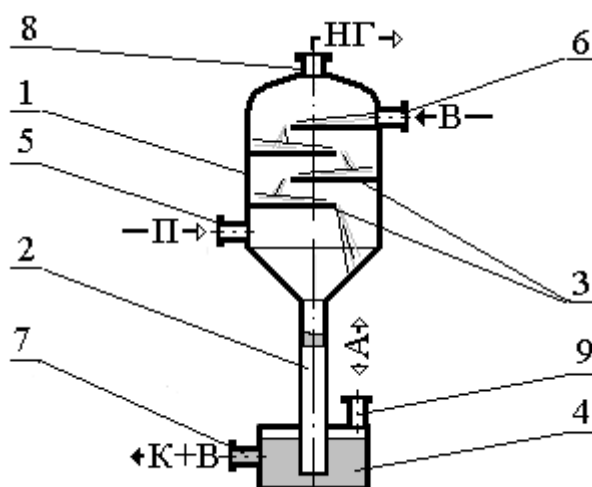
Рис. 8 – Барометрический конденсатор:
