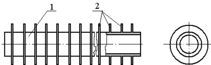
Рис. 6 – Оребренная теплообменная труба: 1 – труба; 2 – ребра
