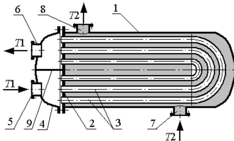
Рис. 3 – Кожухотрубчатый теплообменник с U-образными трубами: 1 – кожух; 2 – трубная решетка; 3 – U-образные трубы; 4 – крышка; 5 и 6 – штуцера трубного пространства; 7 и 8 – штуцера межтрубного пространства; 9 – перегородка в распределительной камере
